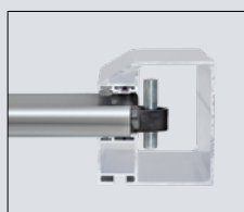
Crochet anti-tempête en acier de série à partir d'une largeur de rideau de 7 500 mm (rideau à lames)
