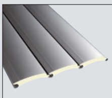
Deco therm S, acier Largeur de rideau max. 7 500 mm, hauteur de rideau 2 500 – 8 500 mm
