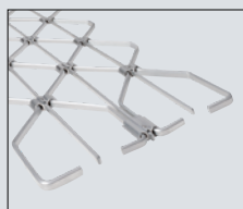
HG-L, aluminium Largeur de rideau / grille max. 6 000 mm, hauteur de rideau / grille max. 4 500 mm
