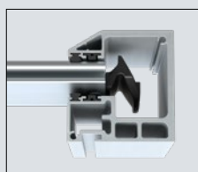
Crochet anti-tempête W4 (rideau à lames)
