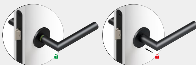
Axialdruck verriegelt | Axialzug entriegelt
