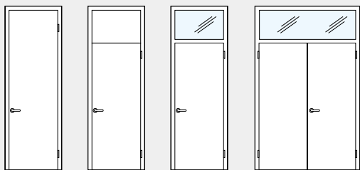
1-flügelig geschosshoch
