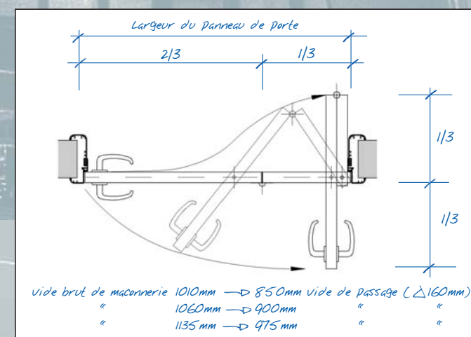
Porte RST Kuffner avec huisserie en aluminium type URS roundline Grâce à son ouverture ergonomique, la porte ne pivote que sur 1/3 de sa largeur totale.
